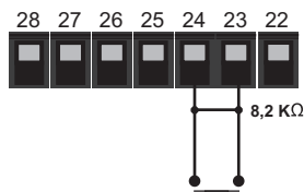
CONNEXION PHOTOCELLULE OUVERTURE (Microswitch n°4 OFF)
