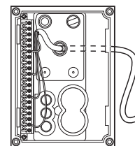
Câblage de commande
