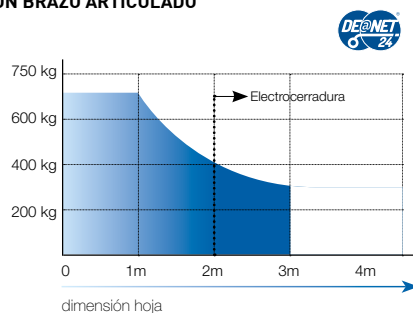
ESQUEMA DE USO CON BRAZO ARTICULADO
