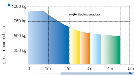
OLI - ESQUEMA DE USO
