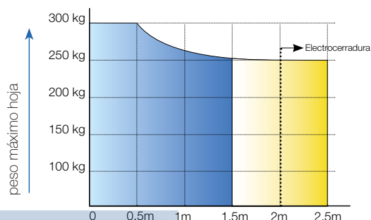
GEKO - ESQUEMA DE USO
