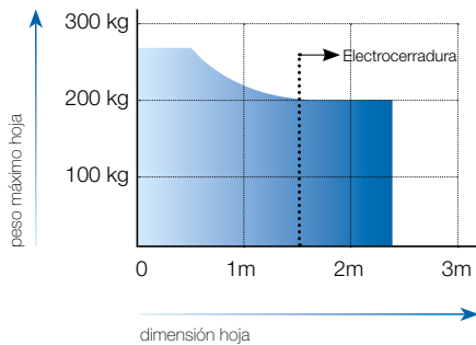
ESQUEMA DE USO CON BRAZO ARTICULADO
