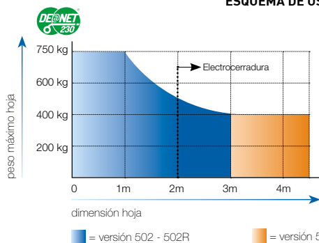
ESQUEMA DE USO CON BRAZO ARTICULADO
