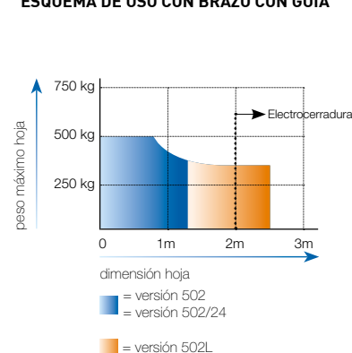
ESQUEMA DE USO CON BRAZO CON GUIA
