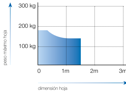
ESQUEMA DE USO CON BRAZO CON GUIA
