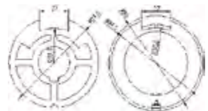
At32 Ø 59 redondo Ø 85mm MT59 / round Ø 85mm MT59 / rond Ø 85mm MT59 / redondo Ø 85mm MT59 Ref.: PATUBU0213
